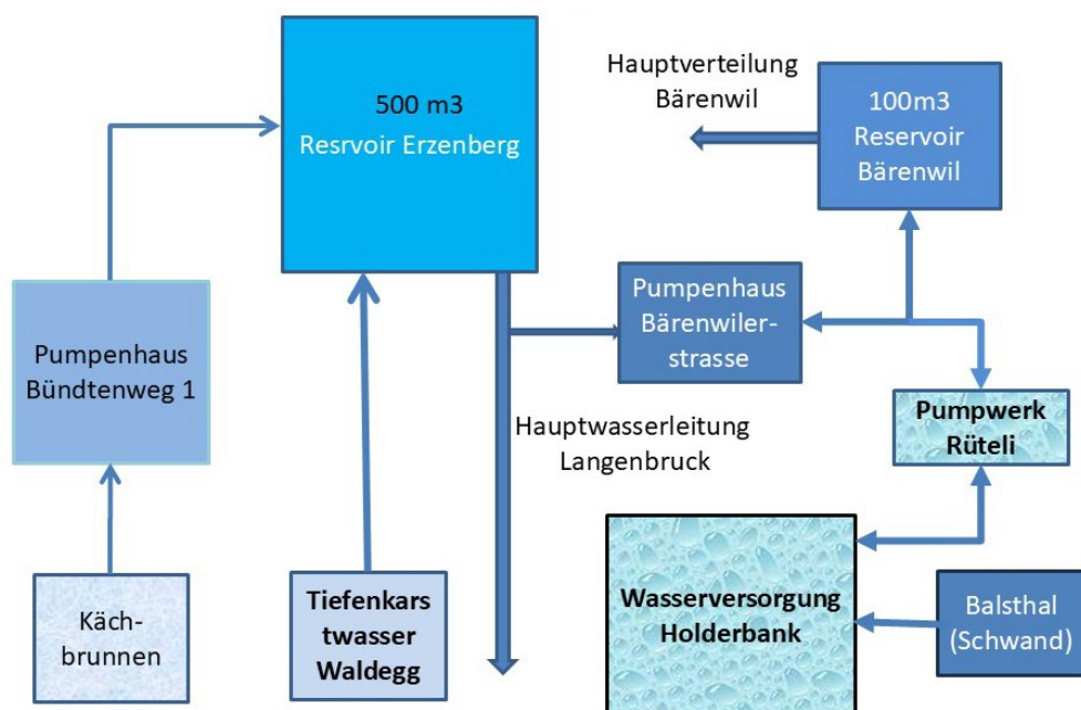
Schema: Wassergewinnung Langenbruck 2026
